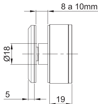
DETALLE DE BARRENO
