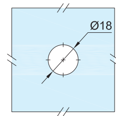
DETALLE DE BARRENO
